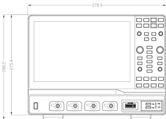
正视图
